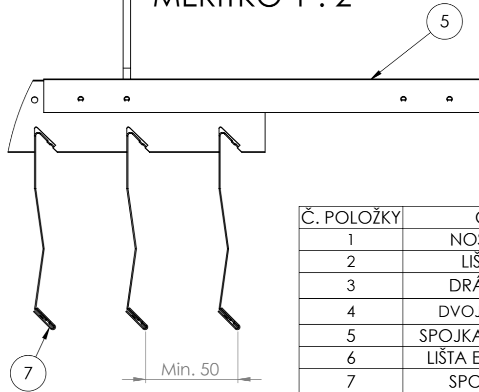
DETAIL A MĚŘITKO 1 : 2
